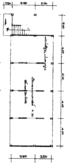
План другого поверху 1:100
