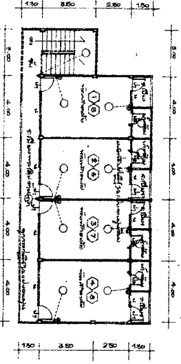
План другого поверху 1:100
